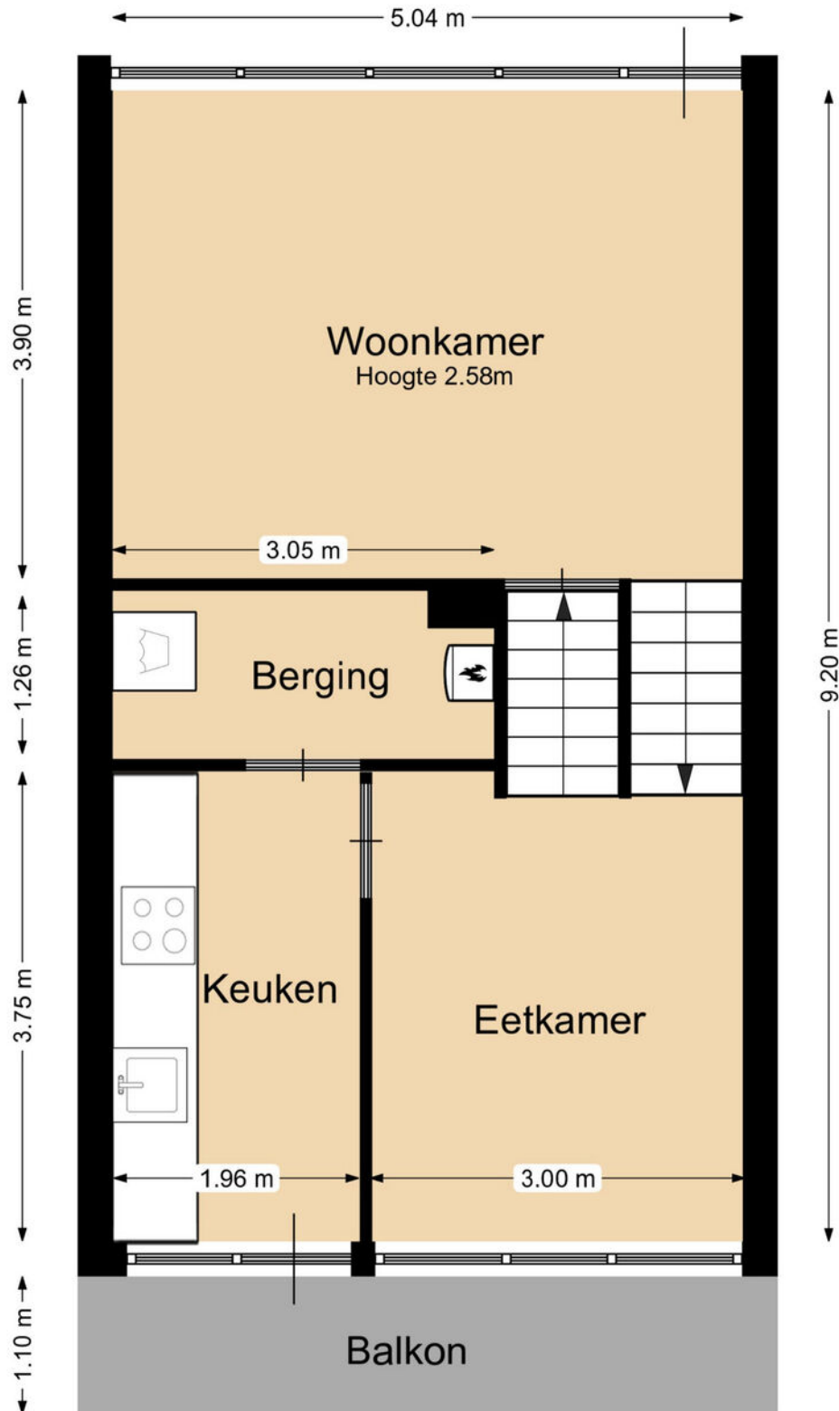
Moeflonstraat 32 Begane grond / 1e verdieping
